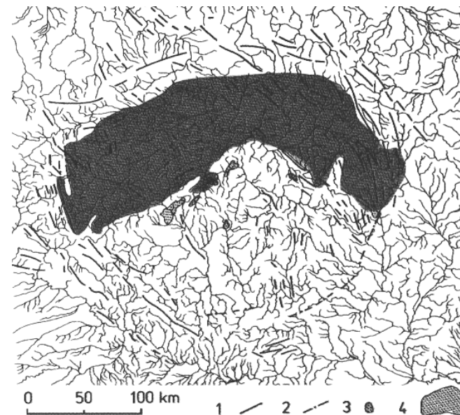
Bildo 17: Pleniĝo en la proterozoiko de la origina kratero.
