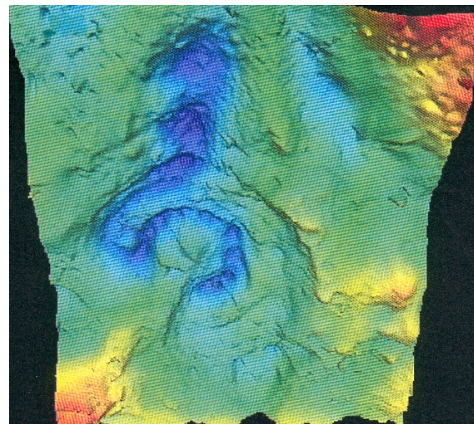
Bildo 3: Gravimetria mapo de la kratero Chicxulub (Grupo de Investigación del Cráter Chicxulub del Instituto de Geofísica de la U.N.A.M.)
