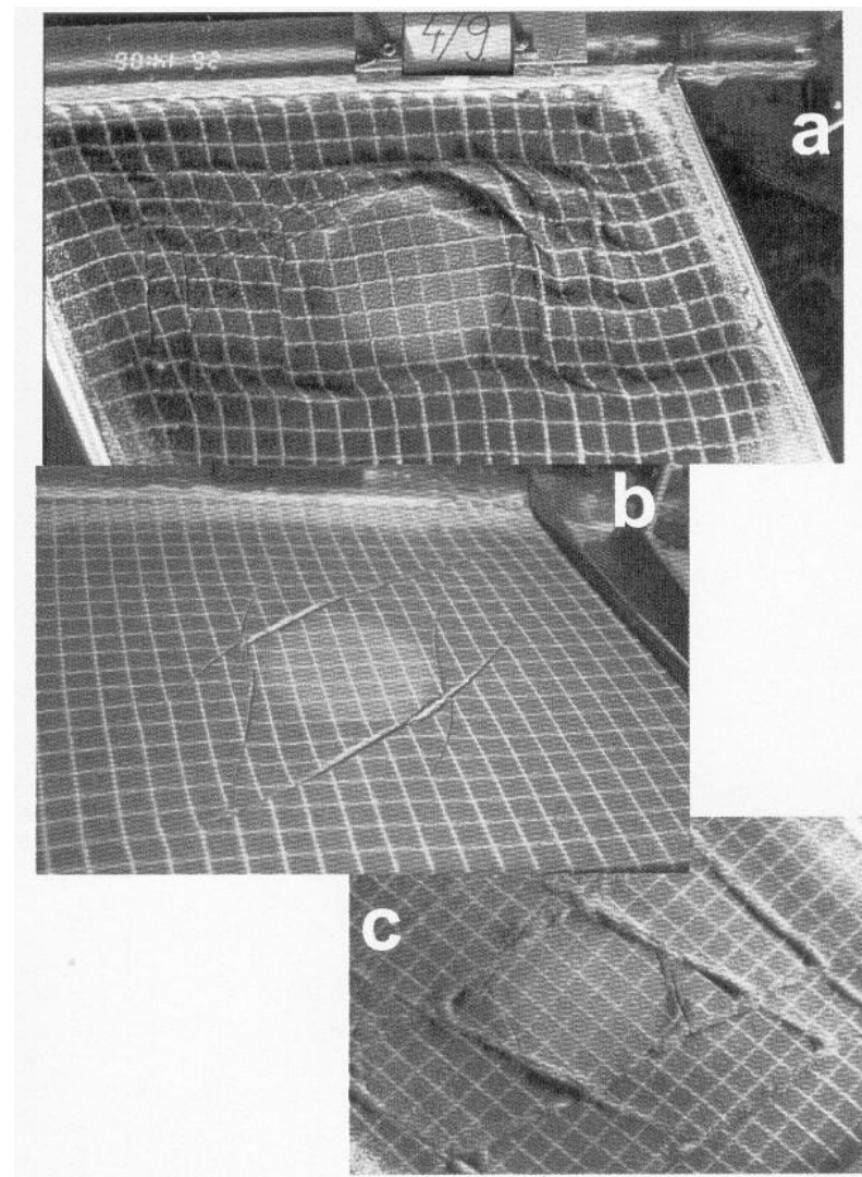
Bildo 18: Analoga modelo kiel formiĝas huffereca strukturo ĉirkaŭ solidigitaj diskoj de la origina kratero, a = formiĝo de huffero en mallarĝa glituzono ĉirkaŭ solida disko, b, c = formiĝo de rombo en pli larĝa glituzono ĉirkaŭ solida disko.
