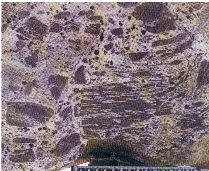
Bildo 5: Origina brekcieca pseŭdotahilit-vejno ("granat"-roko de Taboro)
