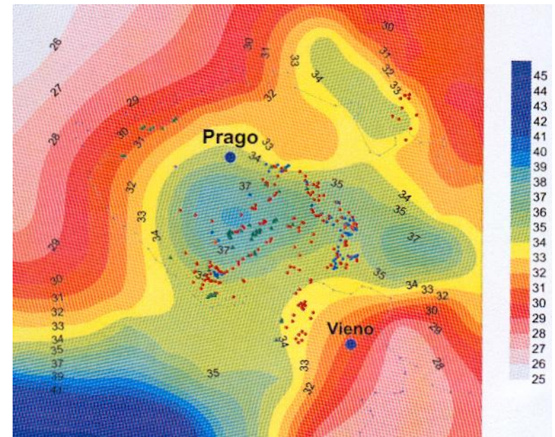
Bildo 14: Kavoj en la Moho-surfaco laŭ Beránek (1979) kaj disvastiĝo de ultrabazajoj, eklogitoj kaj granulit-korpetoj en moldanubiko laŭ Machart (1982) kaj Vrána k.a. (1995).
