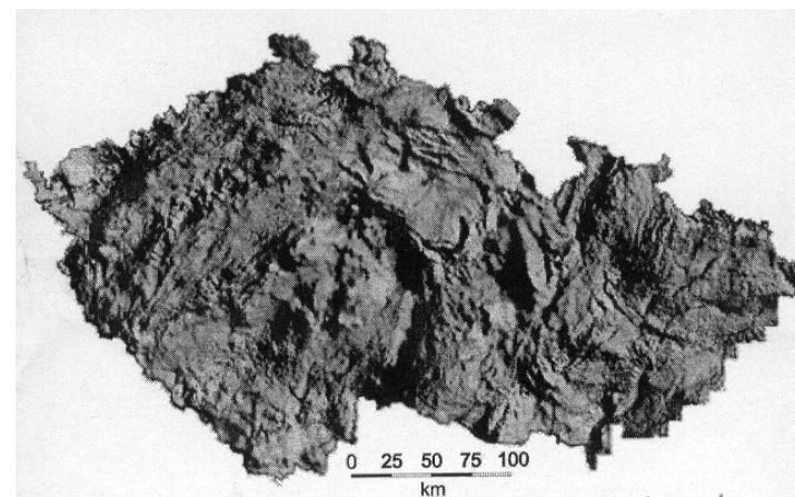
Bildo 2: Gravimetria mapo de la bohemia kratero
