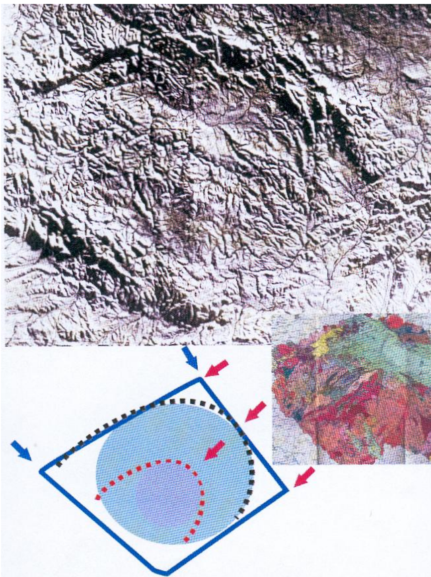
Bildo 19: Nuntempa neopaleozoika ĝis terciara strukturo romba kaj huffera ĉirkaŭ la interna kaj ekstera krater-cirkloj.
