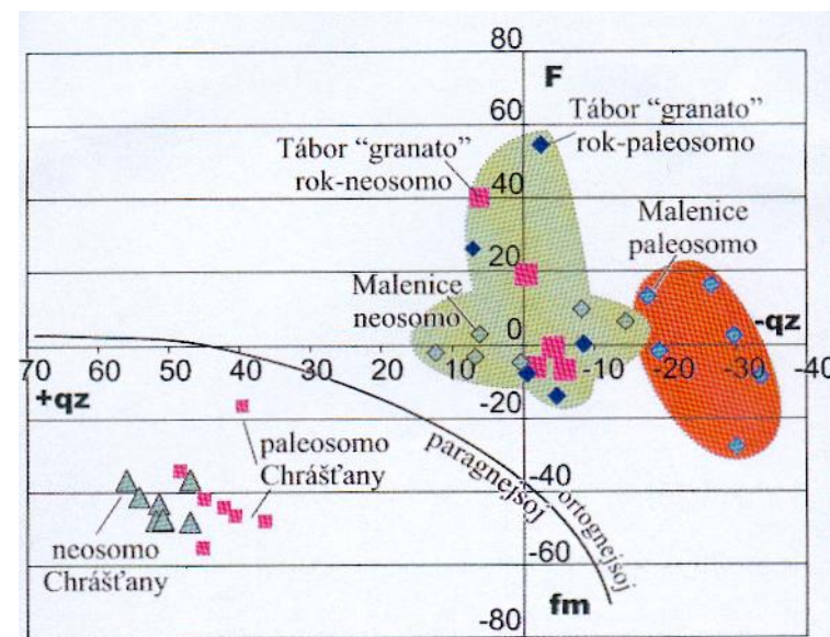
Bildo 6: Ĥemia konsisto de la pseŭdotahilit-vejnoj (grafikaĵo laŭ Köhler-Raaz, 1951)
