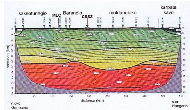
Bildo 13: Seisma profilo Celebration 09 laŭ Hrubcová k.a. (2002). MLC = mariabana komplekso, CBSZ = centraboheemia glituzono.
