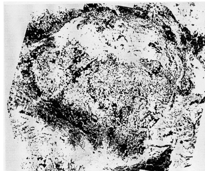
Bildo 1: Satelit-foto de Bohemio
